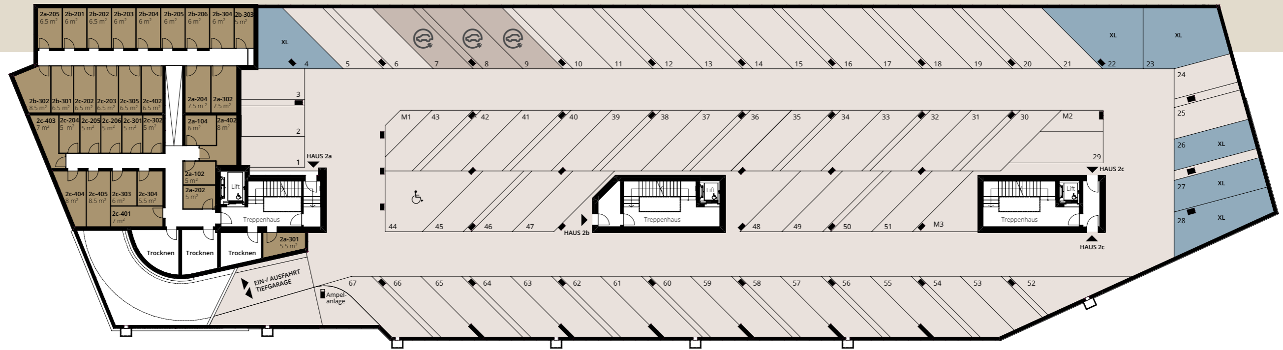
UNTERGESCHOSS
